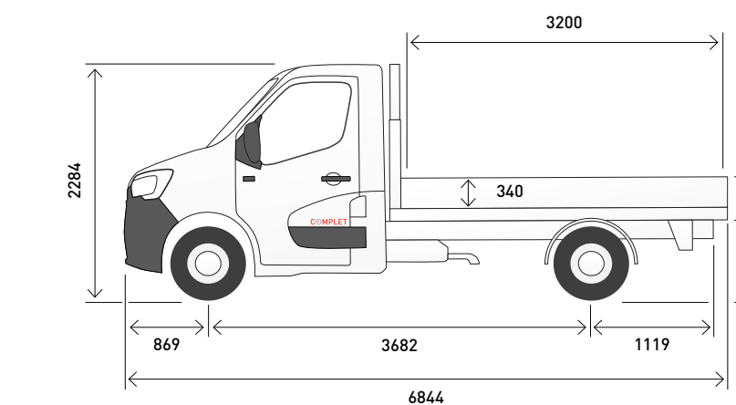
CABINE SIMPLE AVEC BENNE BASCULANTE À 3 CÔTÉS
