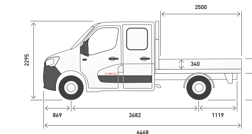
CABINE DOUBLE AVEC BENNE BASCULANTE À 3 CÔTÉS
